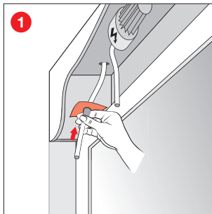
1 Manschette über die Leitung ziehen.
